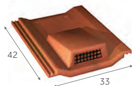
Tuile chatière grillagée (ouverture 25 cm 2 )
