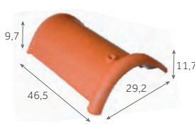
Faîtière/arêtier demi-ronde de 40 ventilée 2,5 au m 4 kg/pièce 144 / palette
