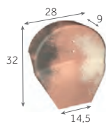
Fronton de rive ronde pour Faîtière conique/demi-ronde de 40 (petit modèle) 3,1 kg/pièce 72 / palette
