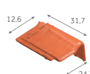
Tuile de rive droite 4,1 au m 3,3 kg/pièce 144 / palette
