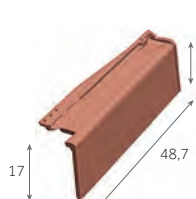
Rive à rabat droite 2,5 au m 3,3 kg/pièce 120 / palette
