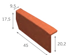
Rive à rabat gauche 2,7 à 3,3 au m 3,7 kg/pièce 90 / palette
