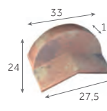
Fronton de rive bardelis de 50 (grand modèle)
