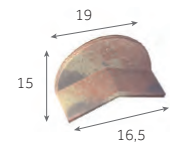
Écusson de rive bardelis demi-ronde de 50
