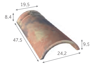
Faitière/arêtier conique de 40
