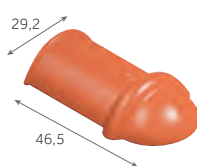
Arêtier d'about demi-rond 3,7 kg/pièce 80 / palette
