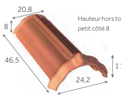
Arêtier à emboîtement de 40
