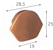
Fronton pour Faîtière/arêtier de 42 à recouvrement
