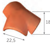
Rencontre 3 voies universelle
