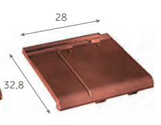
Tuile et demie d'about
