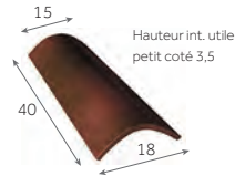
Arêtier tige de botte de 33
