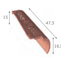
Rive ronde droite 2,7 au m 2,8 kg/pièce 120 / palette
