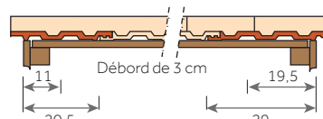
Montage avec tuiles d'about
