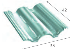
Tuile en verre PLEIN CIEL 4,5 kg/pièce
