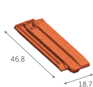
Demi-tuile 2,7 à 3,3 au m 2,4 kg/pièce 192 / palette
