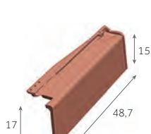
Rive à rabat droite 2,5 au m 3,3 kg/pièce 120 / palette
