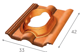
DUROVENT Tuile à douille DOUBLE ROMANE (Ø 110 à 160 mm)
