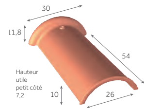
Faîtière demi-ronde de 50 2 au m 5,5 kg/pièce 125 / palette
