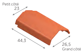
Arêtier à pans de 40 2,5 au m 4,6 kg/pièce 45 / palette
