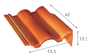
Tuile de rive universelle droite 3,2 au m 7,1 kg/pièce 32 / palette
