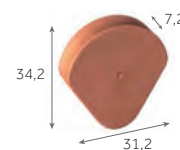
Fronton de rive à rabat pour Faitière demi-ronde 3 kg/pièce 100 / palette
