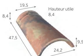
Faîtière/arêtier conique de 40
