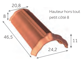
Arêtier à emboîtement de 40
