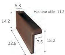
Rive standard gauche 3,7 au m 2 kg/pièce 250 / palette
