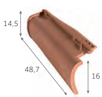
Rive ronde gauche 2,5 au m 3 kg/pièce 120 / palette
