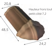
Arêtier d'about à emboîtement de 40 3,3 kg/pièce 90 / palette
