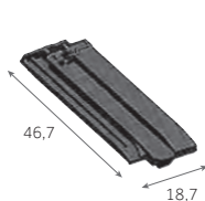
Demi-tuile 2,7 à 3,3 au m 2,4 kg/pièce 192 / palette
