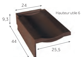
Tuile de rive gauche 2,8 au m 4,5 kg/pièce 80 / palette
