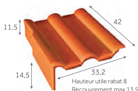
Tuile de rive universelle gauche 3,2 au m 6,6 kg/pièce 32 / palette
