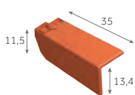
Demi-tuile de rive gauche*
