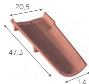
Canal sablière
