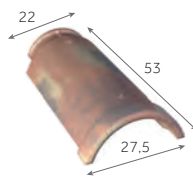
Faitière/arêtier demi-ronde de 50
