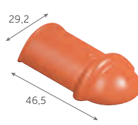
Arêtier d'about demi-rond 3,7 kg/pièce 80 / palette
