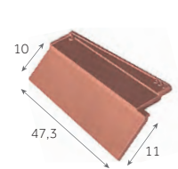
Rive bardelis gauche 2,7 au m 2,1 kg/pièce 140 / palette
