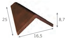
Arêtier cornier
