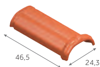
Arêtier ornemental de 40 2,3 au m 3,5 kg/pièce 160 / palette
