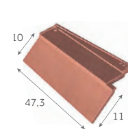
Rive bardelis gauche 2,7 au m 2,1 kg/pièce 140 / palette
