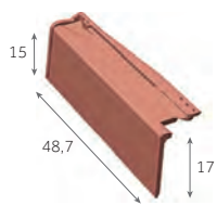
Rive à rabat gauche 2,5 au m 3,3 kg/pièce 120 / palette
