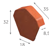
Fronton début/fin pour faîtière à pans 3,6 kg/pièce 40 / palette
