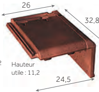
Tuile de rive droite
