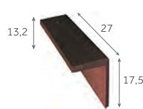
Demi-tuile de rive à rabat droite
