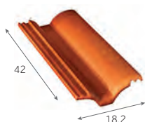
Demi-tuile - 2,3 kg/pièce 120 / palette
