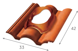
DUROVENT Tuile à douille PLEIN CIEL (Ø 110 à 160 mm)
