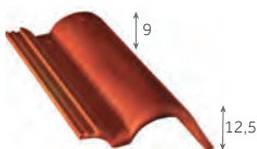
Rive ronde droite 3,2 au m 4,3 kg/pièce 34 / palette
