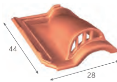
Tuile châtière (ouverture de 21 cm²)
