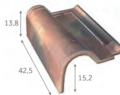
Tuile de rive gauche 2,8 au m 4,5 kg/pièce 48 / palette
