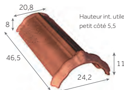
Arêtier de 40 à emboîtement
