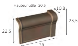
Rive universelle de 33 gauche 3 au m 3,4 kg/pièce 164 / palette
