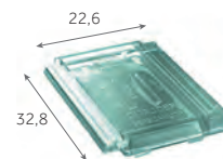
Tuile en verre RÉGENCE/CHARTREUSE 2,3 kg/pièce
