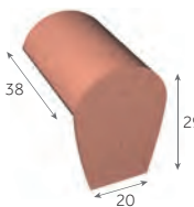
Faîtière d'about conique de 40 (fin)
