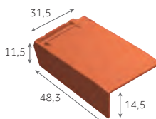
Tuile de rive gauche*
