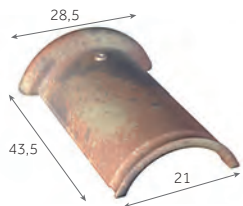
Faîtière demi-ronde de 40 2,5 au m 3,2 kg/pièce 100 / palette
