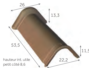
Faîtière de Marseille de 50 (angle 90°) 2 au m 5 kg/pièce 250 / palette
