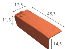
Demi-tuile de rive gauche*
