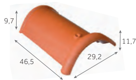
Faîtière/arêtier demi-ronde de 40 ventilée 2,5 au m 4 kg/pièce 144 / palette
