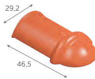
Arêtier d'about demi-ronde 3,7 kg/pièce 80 / palette
