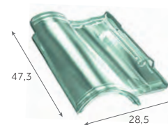
Tuile en verre GALLEANE®12 5,2 kg/pièce
