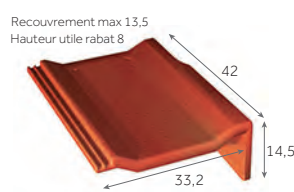
Tuile de rive universelle droite 3,2 au m 6,8 kg/pièce 36 / palette
