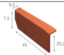
Rive à rabat gauche
