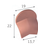
Écusson de rive ronde conique de 40
