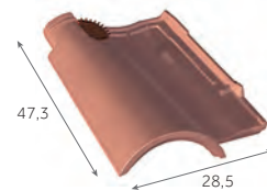
Tuile chatière (ouverture de 16 cm²) 3,4 kg/pièce
