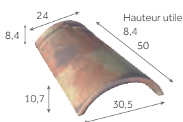
Faîtière/arêteur conique de 50 2,4 au m 4,3 kg/pièce 75 / palette
