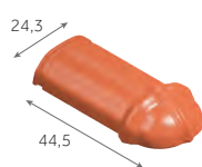
Arêtier d'about ornamental 3,7 kg/pièce
