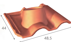
Tuile à douille (Ø int. du tuyau d'évacuation: 175 mm)
