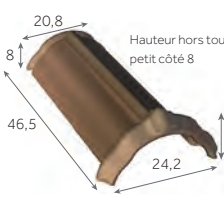
Arêtier à emboîtement de 40 2,5 au m 3,5 kg/pièce 160 / palette
