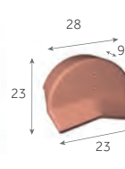
Fronton de rive bardelis de 40 (petit modèle)
