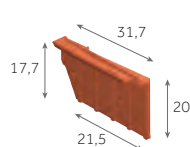
Rive à rabat droite 4,1 au m 2,4 kg/pièce 120 / palette
