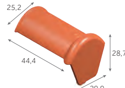
Faîtière d'about demi-ronde (début) 5,2 kg/pièce 24 / palette
