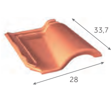
Tuile 3/4 pureau
