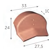
Fronton de rive bardelis de 50 (grand modèle)
