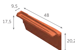
Rive à rabat droit 2,7 à 3,3 au m 3,7 kg/pièce 90 / palette
