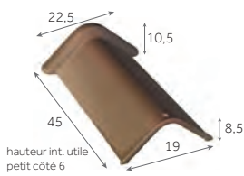
Faîtière de Marseille de 40 (angle 90°) 2,5 au m 3 kg/pièce 240 / palette
