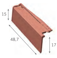
Rive à rabat gauche 2,5 au m 3,3 kg/pièce 120 / palette
