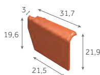
Rive à rabat gauche 4,1 au m 2,5 kg/pièce 120 / palette
