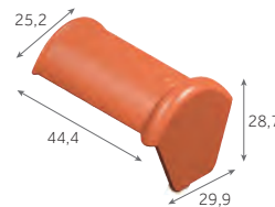
Faîtière d'about demi-ronde (début) 5,2 kg/pièce 24 / palette
