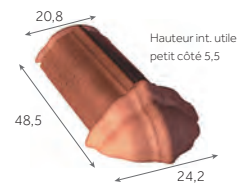
Arêtier d'about à emboîtement de 40
