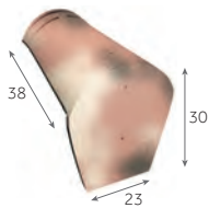
Faîtière d'about conique de 40 (début) 5,1 kg/pièce 48 / palette
