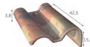
Tuile de rive droite 2,8 au m 5,6 kg/pièce 36 / palette
