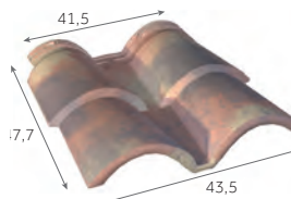
Double tuile 2,4 au m 5,7 kg/pièce 50 / palette
