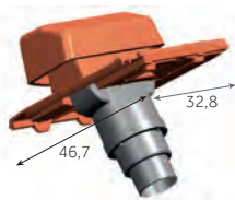
Tuile à douille complète (Ø 100 - 125 - 150 mm Lanterne + adaptateurs plastiques + tuile) 11,4 kg/pièce
