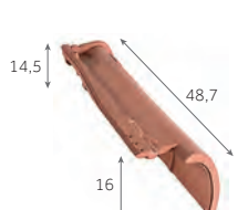
Rive ronde droite 2,5 au m 3,5 kg/pièce 120 / palette
