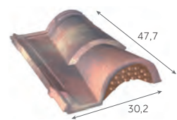
Tuile chatière (ouverture de 16 cm 2 )
