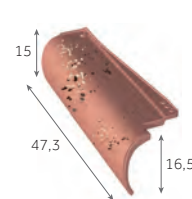
Rive ronde gauche 2,7 au m 2,7 kg/pièce 120 / palette
