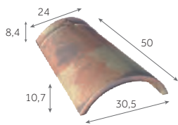
Faitière/arêtier conique de 50
