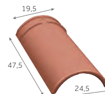
Faîtière/arêtier conique de 40
