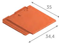
Tuile et demie
