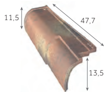
Rive ronde gauche 2,4 au m 2,7 kg/pièce 125 / palette
