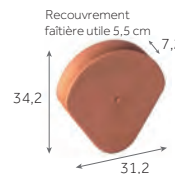
Fronton de rive à rabat pour Faîtière demi-ronde 3 kg/pièce 100 / palette
