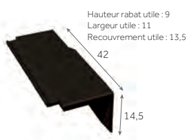
Demi-tuile de rive universelle droite*
