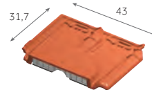
Tuile châtière grillagée (ouverture 31 cm 2 ) 4,1 kg/pièce
