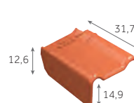
Tuile de rive gauche 4,1 au m 3,4 kg/pièce 144 / palette
