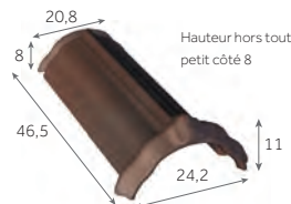
Arêtier d'emboîtement de 40
