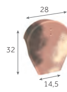
Fronton de rive à rabat pour Faîtière conique/demi-ronde de 40 (petit modèle) 3,1 kg/pièce 72 / palette
