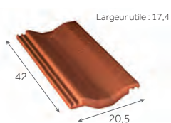
Demi-tuile 3,2 au m 2,9 kg/pièce 120 / palette
