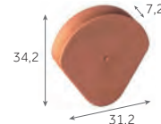
Fronton de rive à rabat pour Faîtière demi-ronde 3 kg/pièce 100 / palette
