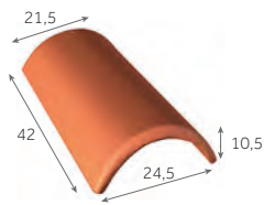
Faîtière/arêtier de 42 à recouvrement
