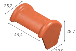
Faîtière d'about demi-ronde (fin) 5,8 kg/pièce 24 / palette
