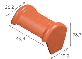
Faitière d'about demi-ronde (fin) 5,8 kg/pièce 24 / palette
