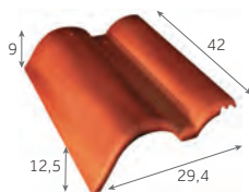
Rive ronde gauche 3,2 au m 4,3 kg/pièce 34 / palette
