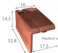
Demi-tuile de rive gauche*
