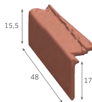
Rive à rabat gauche
