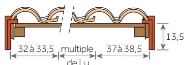
Montage avec rives à rabat et doubles tuiles
