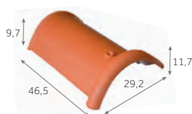
Faîtière/arêtier demi-ronde de 40 ventilée 2,5 au m 4 kg/pièce 144 / palette
