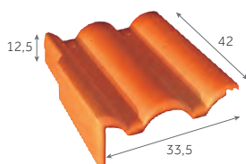
Tuile de rive universelle gauche 3,2 au m 7,4 kg/pièce 32 / palette
