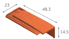
Demi-tuile de rive droite*
