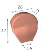
Fronton de rive ronde de 40 (petit modèle)
