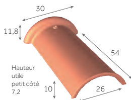
Faîtière demi-ronde de 50
