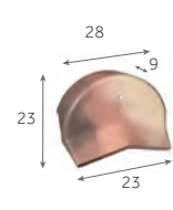
Fronton de rive bardelis de 40 (petit modèle)
