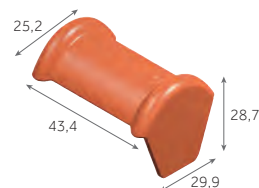
Faîtière d'about demi-ronde (fin) 5,8 kg/pièce 24 / palette
