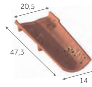
Canal sablière 4 au m 2,1 kg/pièce 150 / palette
