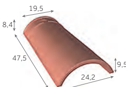
Faîtière/arêtier conique de 40 (selon coloris)
