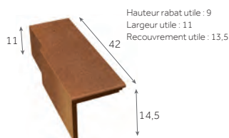
Demi-tuile de rive universelle gauche*
