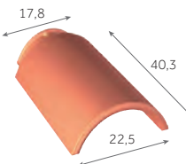
Faîtière/arêtier à emboîtement de 33
