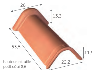
Faîtière de Marseille de 50 (angle 90°) 2 au m 5 kg/pièce 200 / palette
