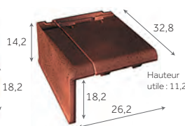
Tuile de rive gauche
