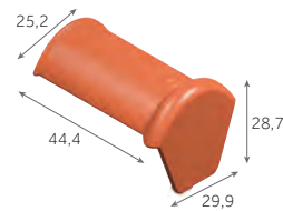
Faitière d'about demi-ronde (début) 5,2 kg/pièce 24 / palette
