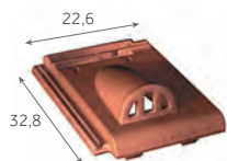
Tuile chatière grillagée (ouverture de 13 cm²)
