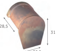
Faitière d'about demi-ronde de 50 (fin)
