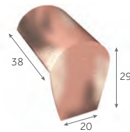
Faîtière d'about conique de 40 (fin) 5,1 kg/pièce 48 / palette
