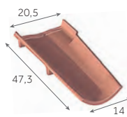
Canal sablière 4 au m 2,1 kg/pièce 160 / palette
