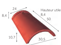
Faîtière/arêtier conique de 50
