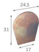
Écusson de 50
