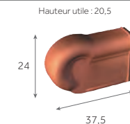
About de rive de 33 droite**
