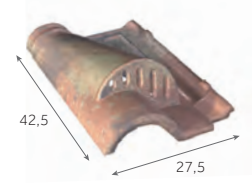
Tuile chatière grillagée (ouverture de 20 cm²) 3,5 kg/pièce
