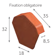
Fronton pour Faîtière à pans (début/fin) 3,6 kg/pièce 40 / palette
