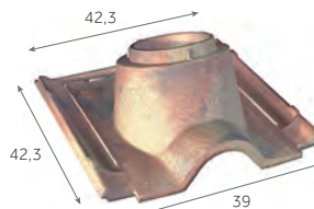
Tuile à douille (Ø int. du tuyau d'évacuation : 150 mm) 5,8 kg/pièce
