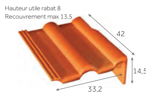
Tuile de rive universelle droite 3,2 au m 6,6 kg/pièce 32 / palette
