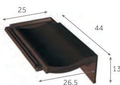
Tuile de rive droite 2,8 au m 4,5 kg/pièce 80 / palette
