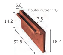
Rive à rabat droite*
