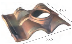
Tuile à douille (Ø int. du tuyau d'évacuation: 150 mm)
