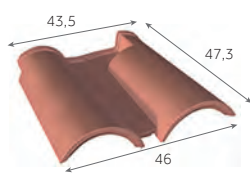
Double tuile (tuile de raccordement) 2,7 au m 6,2 kg/pièce 40 / palette
