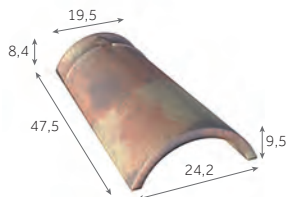
Faîtière/arêtier conique de 40 2,6 au m 3,3 kg/pièce 100 / palette
