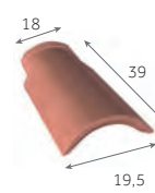
Canal couvert 3/4 de pureau 4 au m 2 kg/pièce 150 / palette
